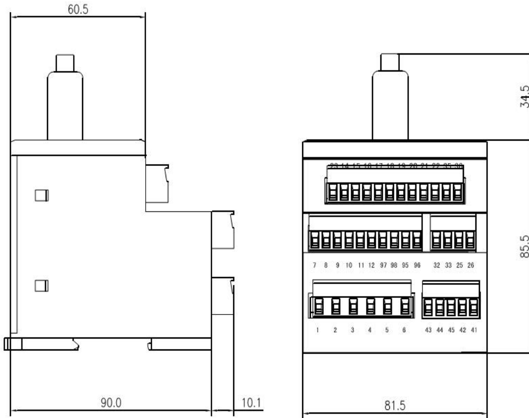
主视图
