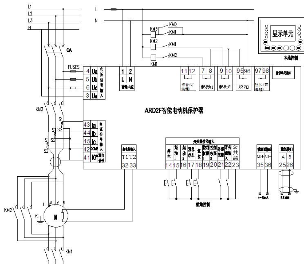
ARD2F 电动机保护器 Y-△启动模式接线图（适用于 1.6、6.3、25、100、250、800A 电流规格）：
