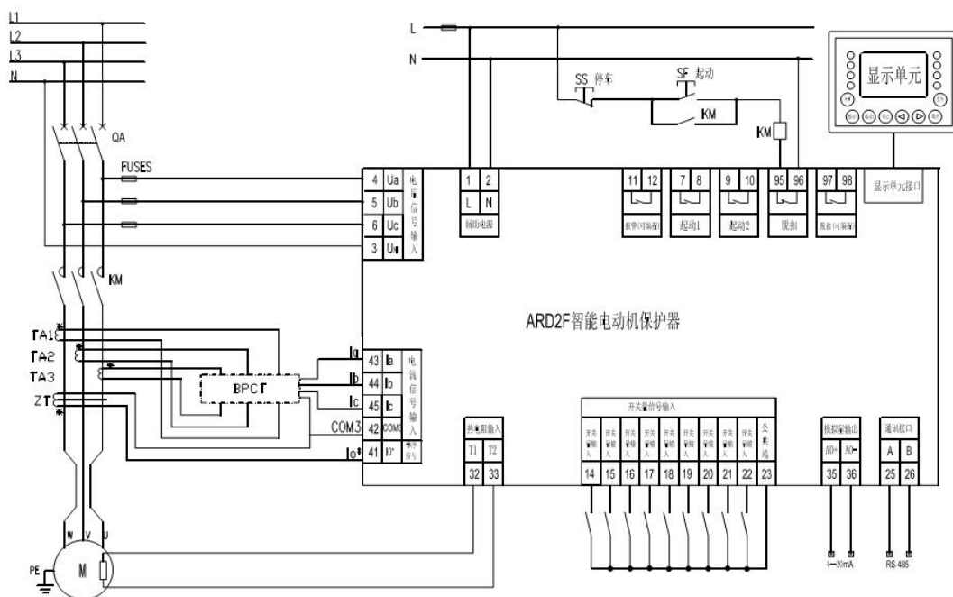
ARD2F 电动机保护器 1A、5A 规格的接线图：
