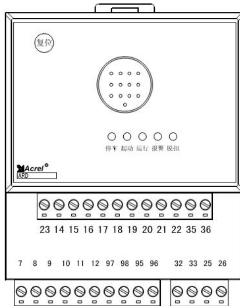
俯视图
